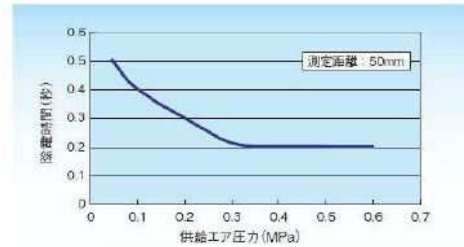
除電特性 [除電時間-供給エア圧力]
