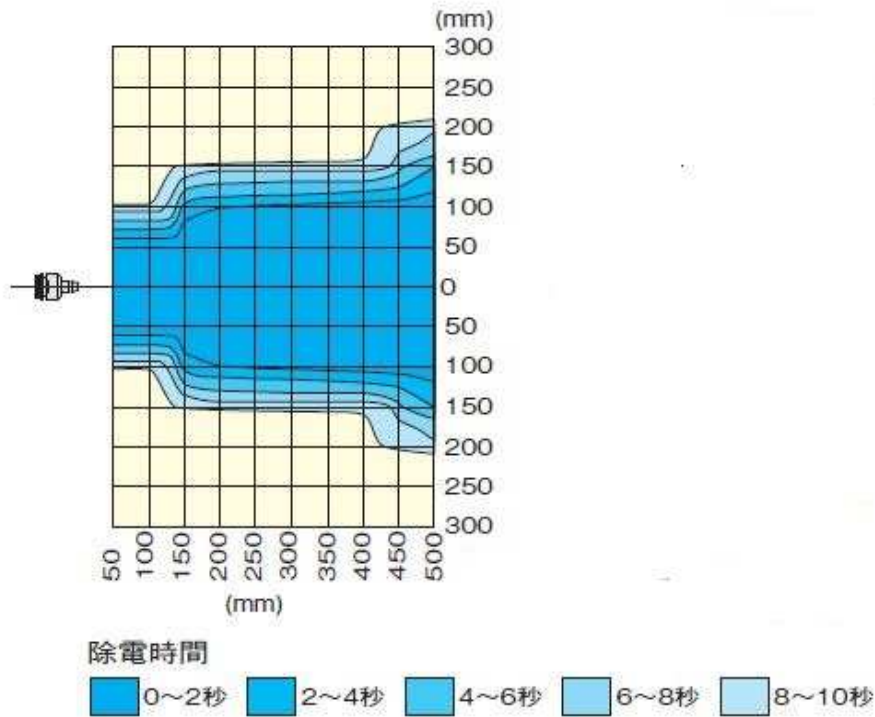
除電特性 [距離-除電時間]
